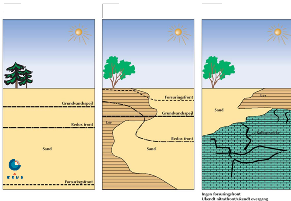
Figur 13. Principskitse over beliggenheden af forsuringssfronten og redoxfronten i tre typiske geologiske situationer: 1) Vestdanmark, hvor jordlagene overvejende består af sand, 2) Østjylland, Fyns og Vestsjælland, hvor geologisk heterogenitet med vekslende ler og sand giver store lokale variationer i dybden til fronterne og 3) områder med kalklag, se Figur 8, hvor sprækkedannelser gør fastlæggelse af nitratfronten i selve kalklagene svær at forudsige. Bemærk, at forsuringssfronten kan ligge både over og under redoxfronten.
